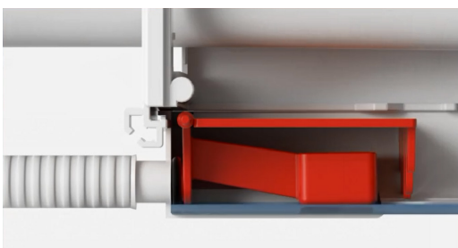
Détail du système de flotteur
