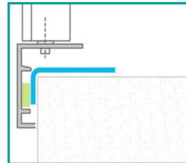
MONTAGE AIMANTS
