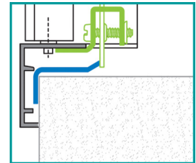
MONTAGE BATTEUSES
