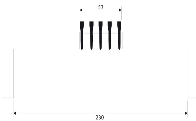
KPW 4 FENTES
