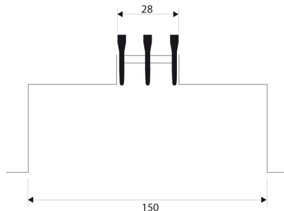
KPW 2 FENTES
