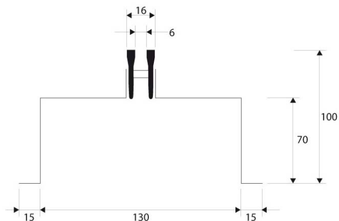
KPW 1 FENTE
