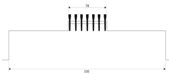
KPW 6 FENTES
