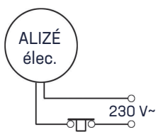
Bouton poussoir normalement fermé
