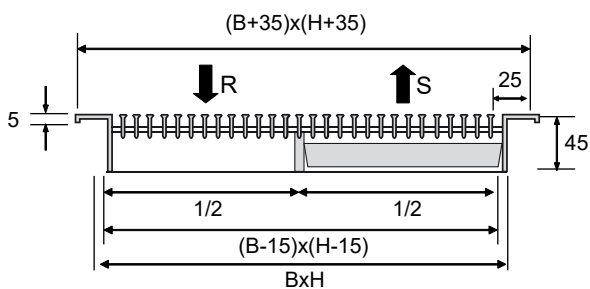
KBL 20/21 S/R SOUFFLAGE CÔTÉ
