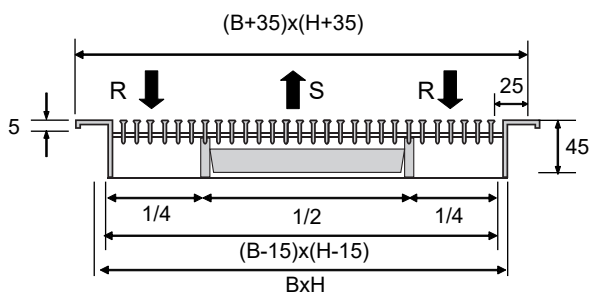
KBL 20/21 S/R SOUFFLAGE CENTRAL
