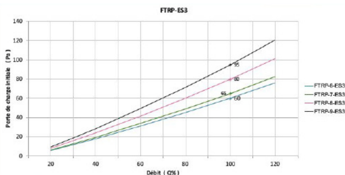
DIAGRAMME DÉBIT / PERTE DE CHARGE
