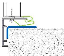
MONTAGE CLIPS
