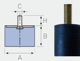
Butée Type D
