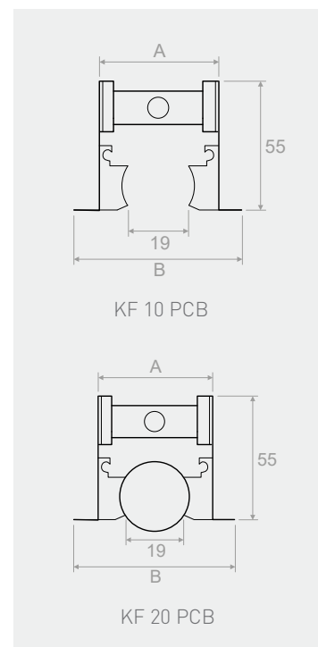
Fixation du plénum avec étriers CVL-CB
