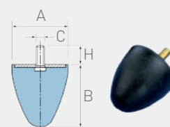
Butée progressive AT
